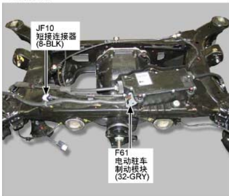
185.后悬架
